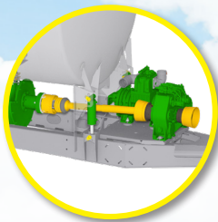
Pompy próżniowe lub Vacu-Storm o dużej wydajności (przepływomierz w opcji)
